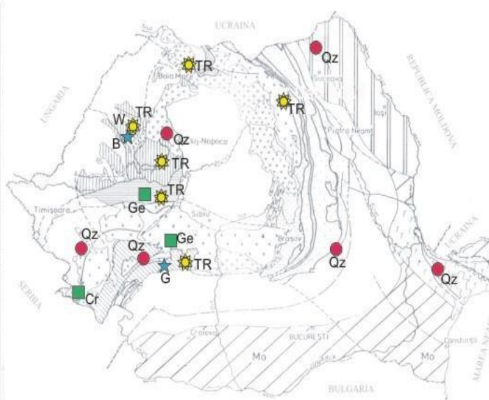
RESURSE POTENȚIALE DE MATERII PRIME CRITICE ÎN ROMÂNIA
