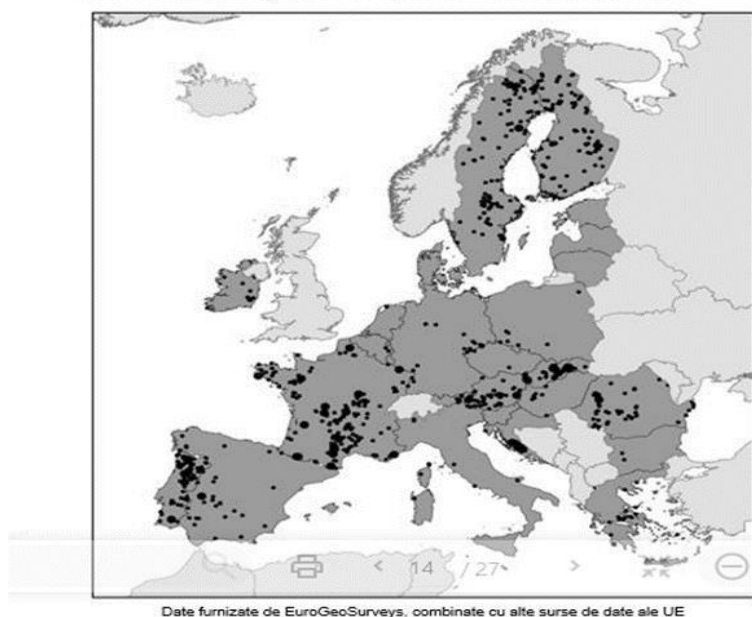
RESURSE POTENȚIALE DE MATERII PRIME CRITICE ÎN UE
